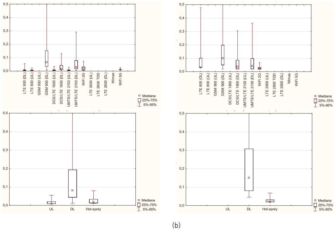
Rycina 1. Ewolucja charakterystyki narażenia na pole-EM emitowane przez urządzenia sieci radiokomunikacyjnych zaobserwowana w typowej galerii handlowej: a) wyniki pomiarów z 2018 r.; b) wyniki pomiarów z 2023 r.; zilustrowano pasma częstotliwości, w których współczynnik RW > 0,01
